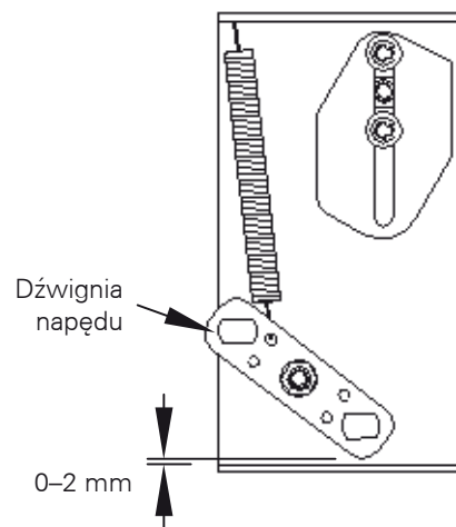
Wyłącznik otwarty rys. 1
