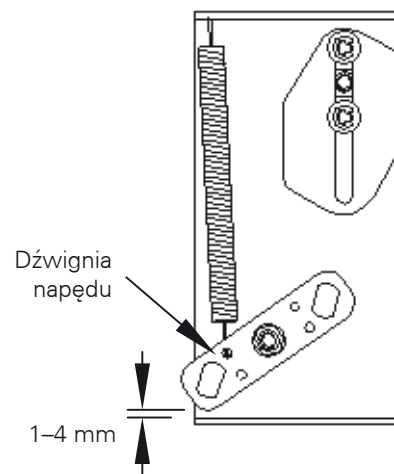
Wyłącznik zamknięty rys. 2
