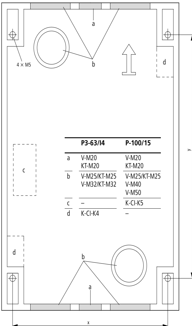
P3...63/I4 P3...100/I5
